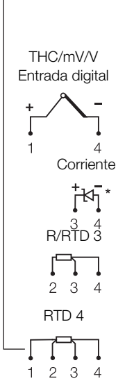
ABCD Una sola entrada
