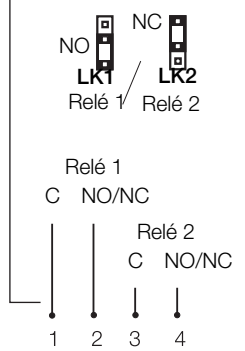
D Relé doble
