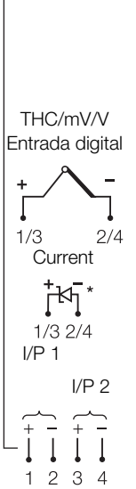
BCD Entrada doble
